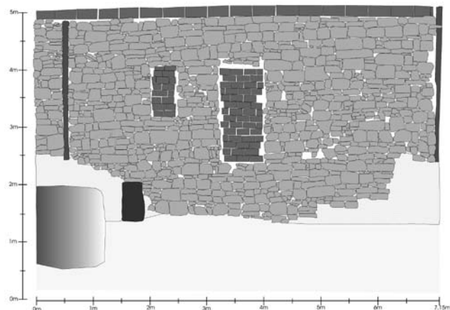
Dibuix en alçat de la muralla del raval de Sant Pere. Autor: Xavier Aguelo, Arqueolític Terra Sub SL.
